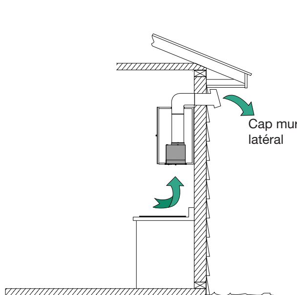
VENTILATION HORIZONTALE AU MUR
