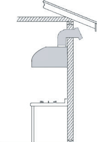
VENTILATION HORIZONTALE AU MUR
