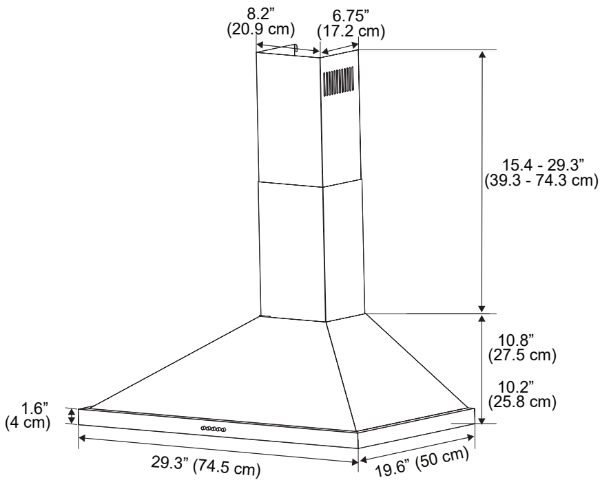
Dimension of: OV-2005 / OV-2007WH / OV-2031 / OV-2020
